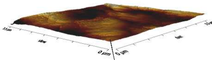
صورة (2) مورفولوجيا غشاء النشأ النانوي المحضر بتركيز 1.5% باستعمال مجهر القوى الذرية
