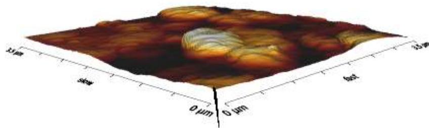
صورة (2) مورفولوجيا غشاء النشأ النانوي المحضر بتركيز 0.5% باستعمال مجهر القوى الذرية
