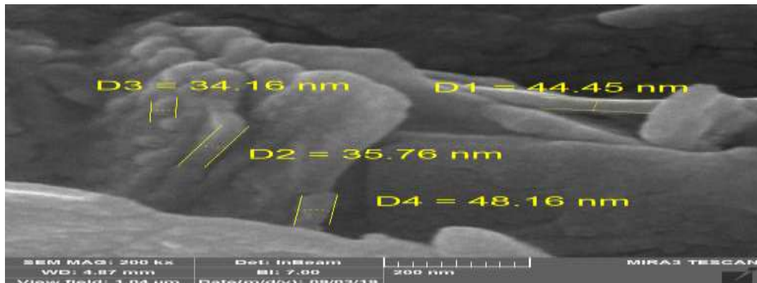
صورة(1) حجم النشا النانوية المحضر باستعمال مجهر المسح الالكتروني
